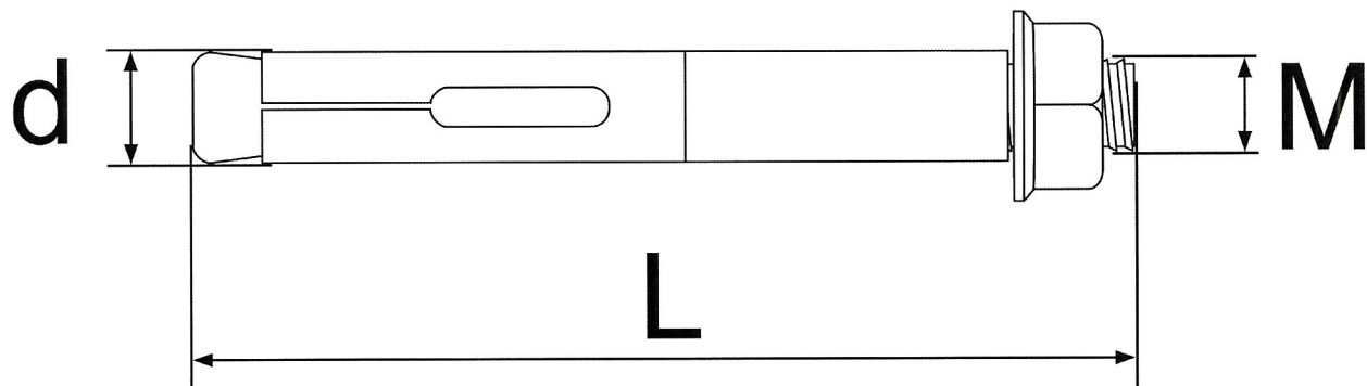
Rysunek A1. Łącznik rozporowy KHA
