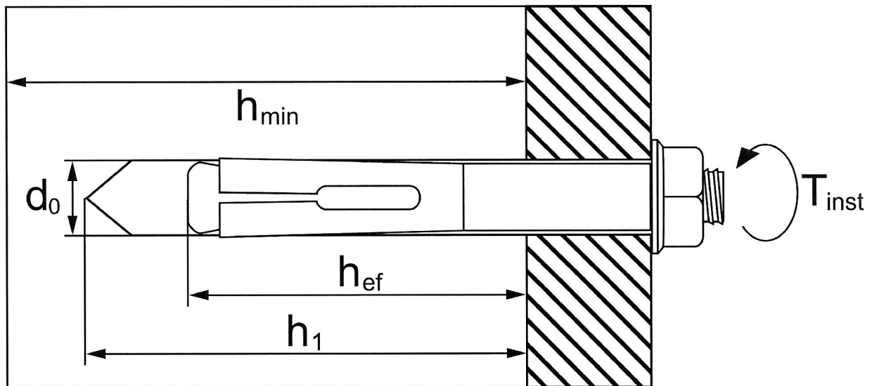
Rysunek B1. Parametry montażowe łączników rozporowych
