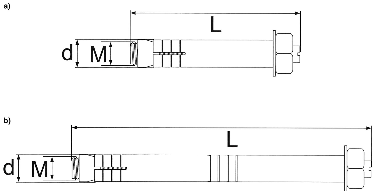
Rysunek A3. Łącznik rozporowy SLR
