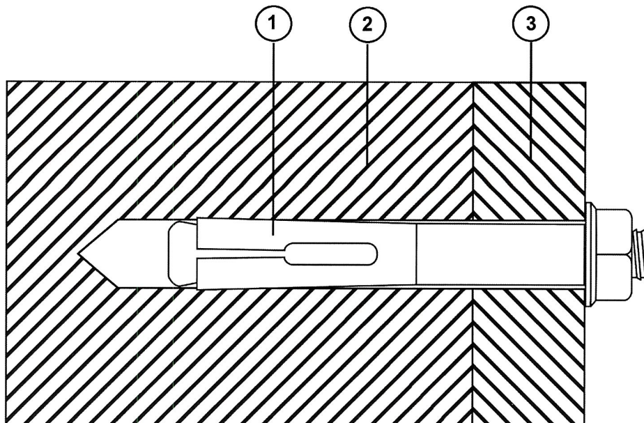
Rysunek A4. Mocowanie z zastosowaniem łącznika rozporowego KHA 1 – łącznik rozporowy, 2 – podłoże, 3 – mocowany element
