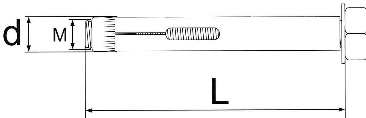
Rysunek A2. Łącznik rozporowy KHA-S
